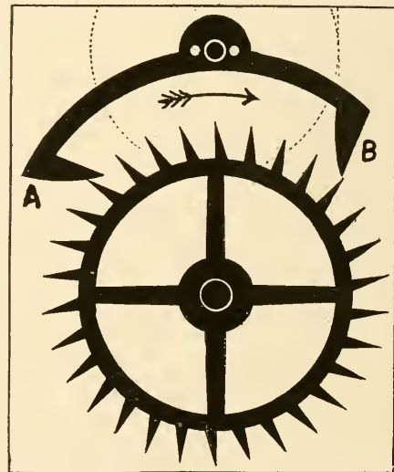
Fig. 27—Anchor Escapement
