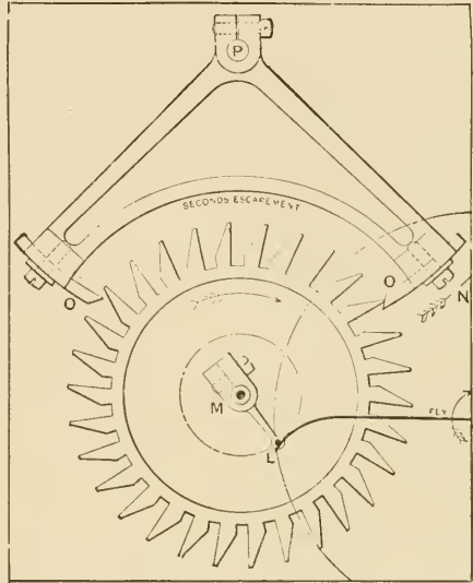
Fig. 29—Dead Beat Escapement
