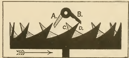
Fig. 25—Verge Escapement
